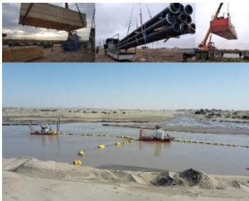
圖片說明：（上）被拆解的挖泥船部件即將踏上 7000 公里的旅途；（下）挖泥船正在阿姆河上作業。（來源：Gebrüder Weiss）
